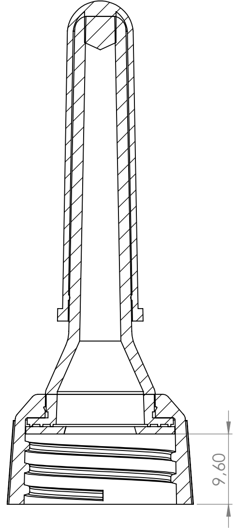
KESIT R-R ÖLÇEK 2 : 1
