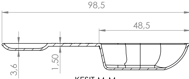
İKESİT M-M ÖLÇEK 1 : 1
