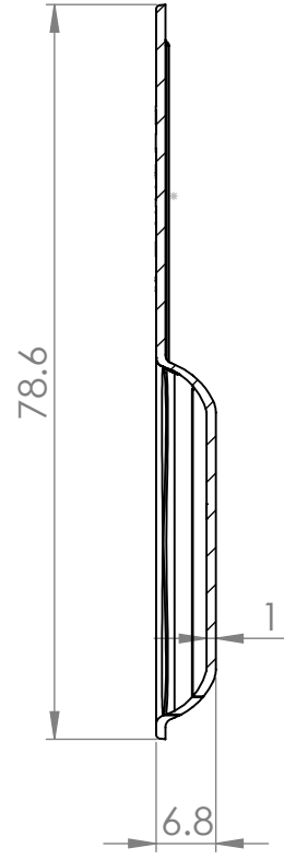
KESİT F-F
