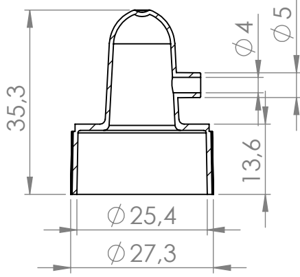
KESİT F-F ÖLÇEK 1 : 1
