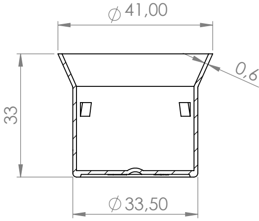
KESİT Q-Q
