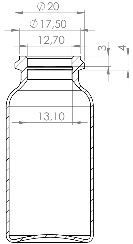
İKESİT M-M ÖLÇEK 3 : 2
