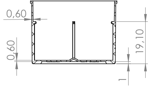
KESIT O-O
